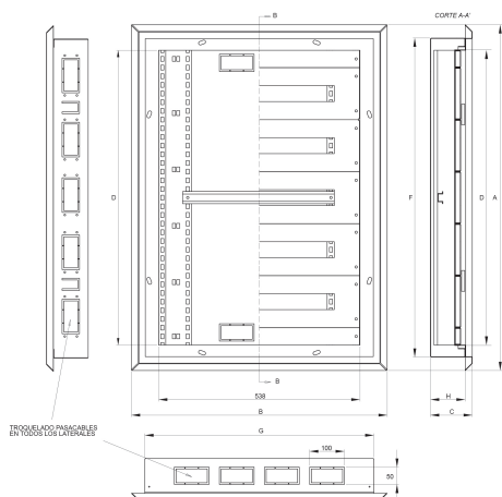
Plano Genérico
